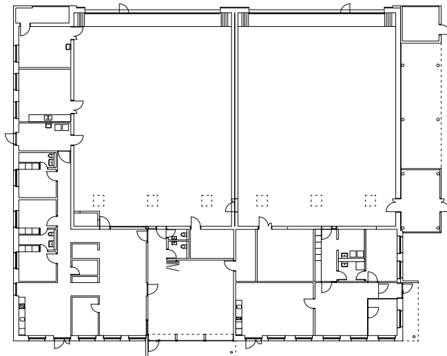
Erdgeschoss Rega
